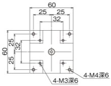
ステージ上面図
