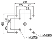
ステージ上面図
