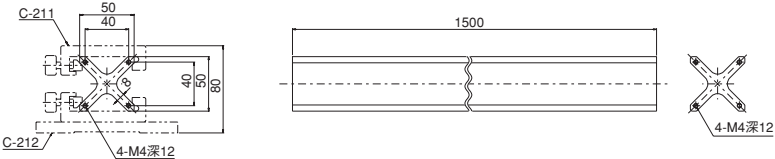
レール、レールキャリアおよびレールスタント'組み合わせ図
