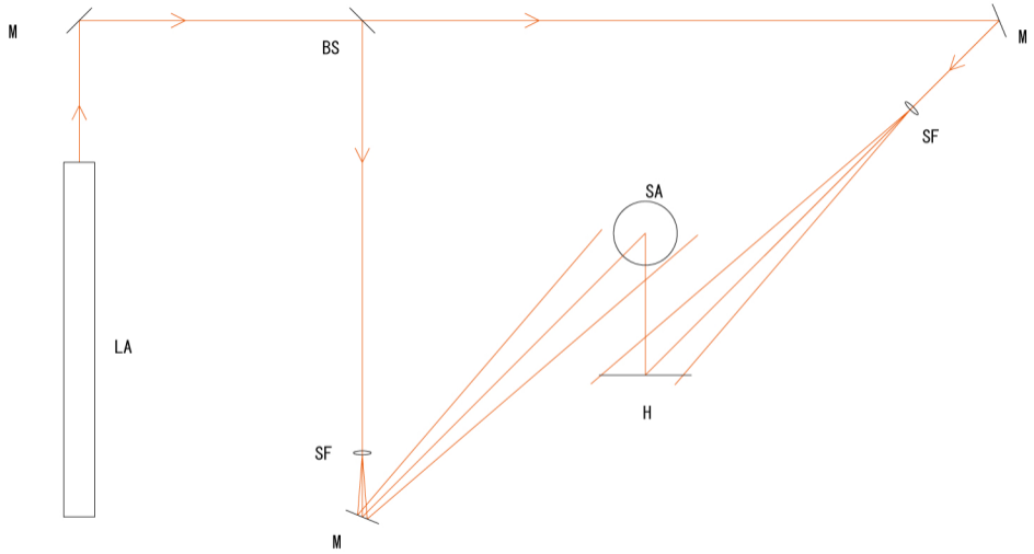
フレネルホログラフィ 光学系
