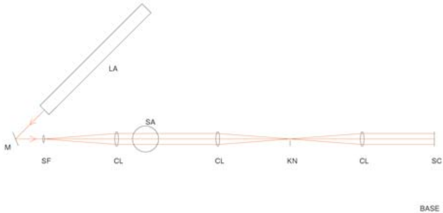
シュリーレン光学装置 光学系
